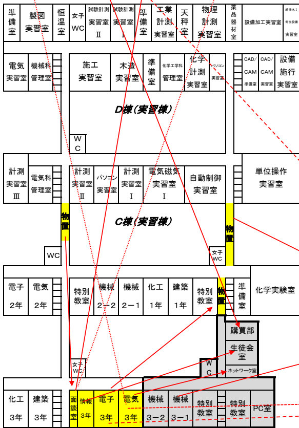
二階平面図
