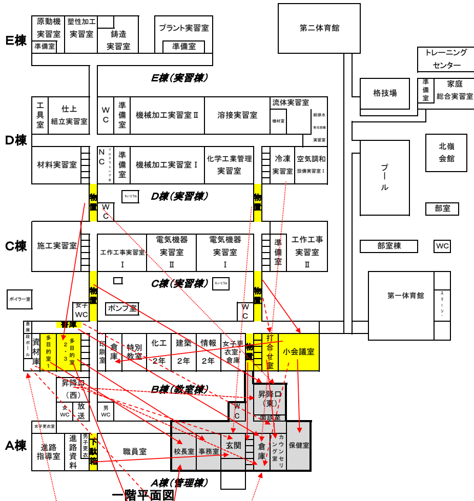
一階平面図
