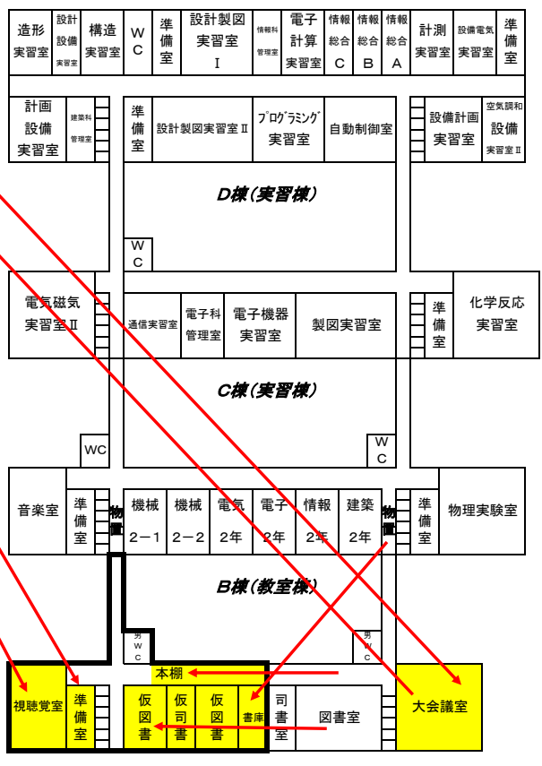
三階平面図
